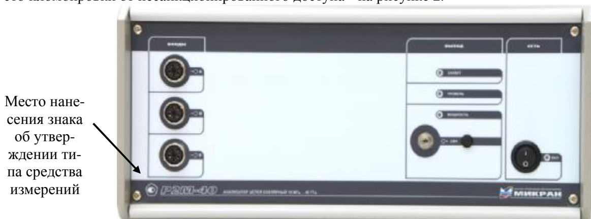
Рисунок 1 – Внешний вид анализаторов цепей скалярных P2M-40
